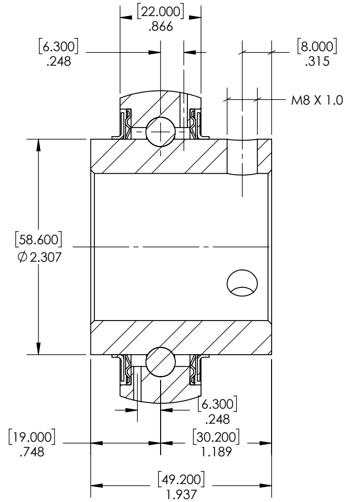
SECTION A-A
